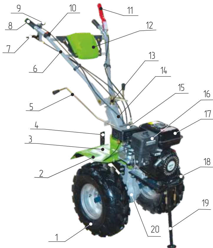
Рис.1 Мотоблок (общий вид)
